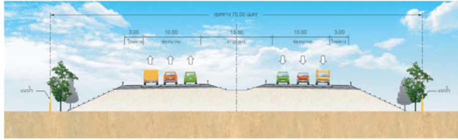
รูปแบบถนน ขนาด 6 ช่องจราจร
